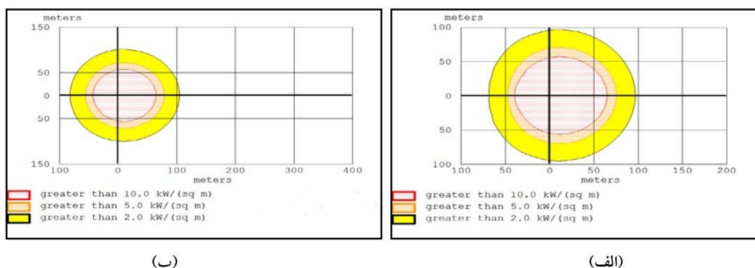
شکل (۲-الف) - مناطق مورد تهدید آتشسوزی متانول بر حسب مسافت در فصل گرم، (ب) مناطق مورد تهدید آتشسوزی متانول بر حسب مسافت در فصل سرد در نمافزار ALOHA
